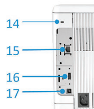
Gros plan des ports d'E/S
